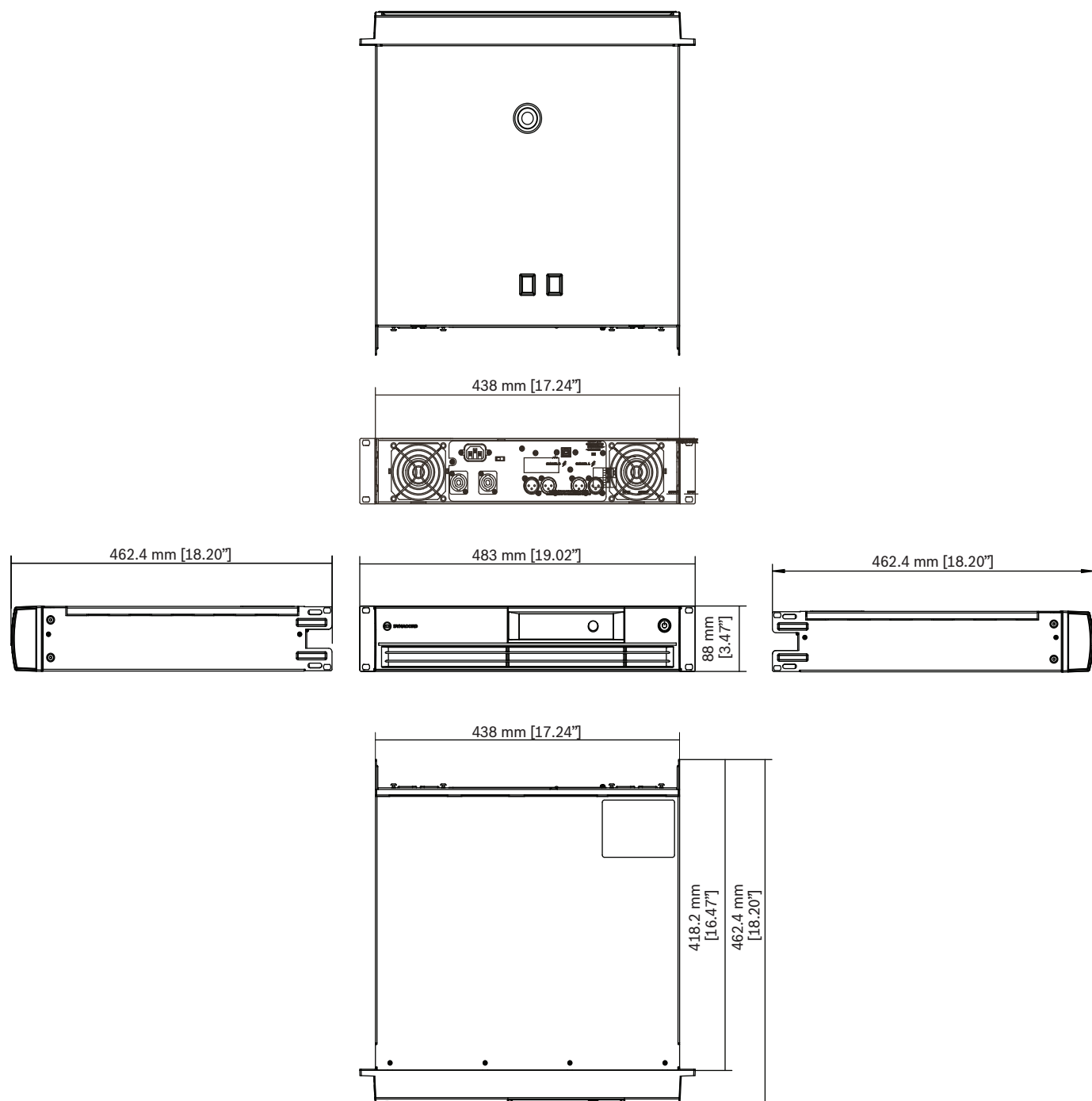
Рис. 1: Размеры
