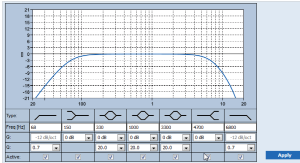
F: Frequenz, G: Verstärkung, Q: Qualitätsfaktor
