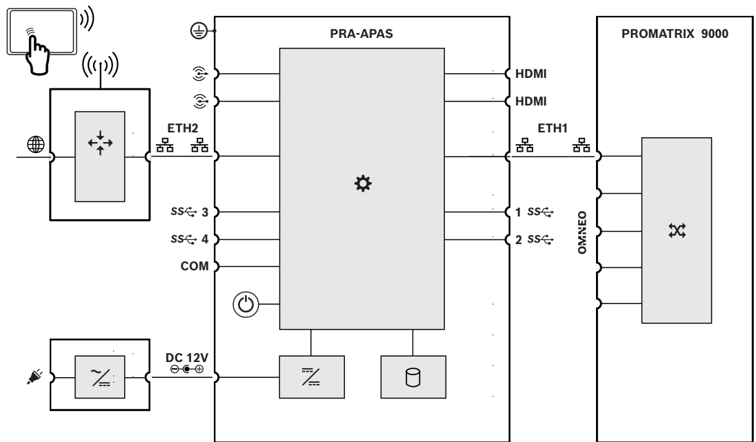
Anschluss- und Funktionsdiagramm
