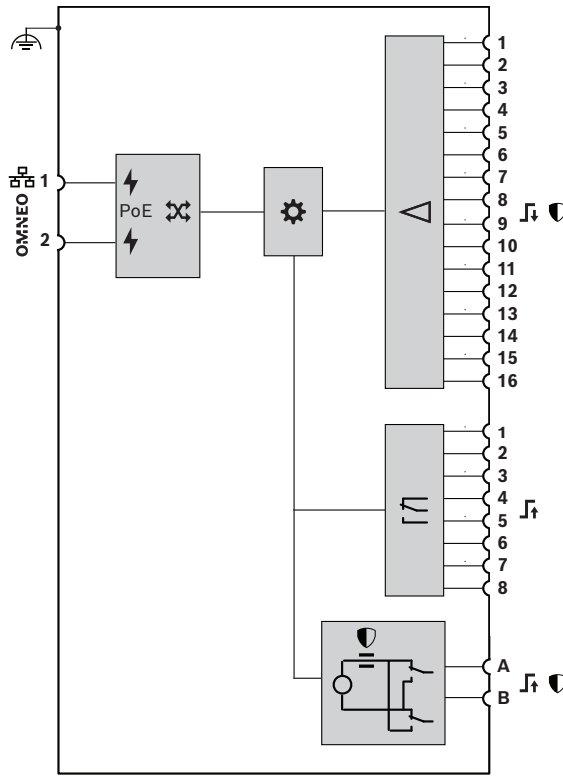
Funktions- und Anschlussdiagramm
