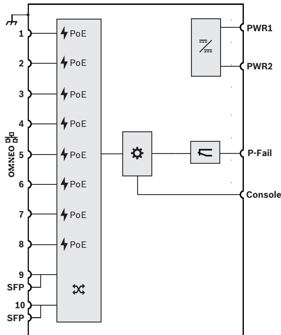
Funktions- und Anschlussdiagramm
