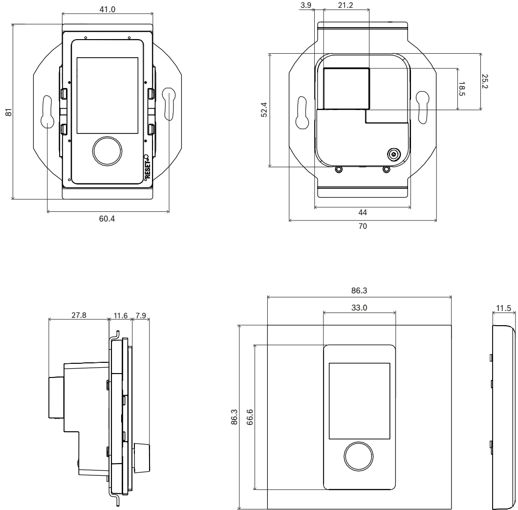
PRA-WCP-EU Wandbedienfeld, EU-Stil
