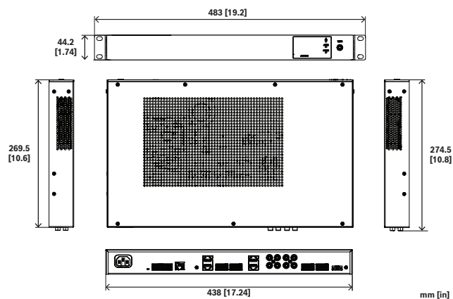
Abb. 1: Maße
