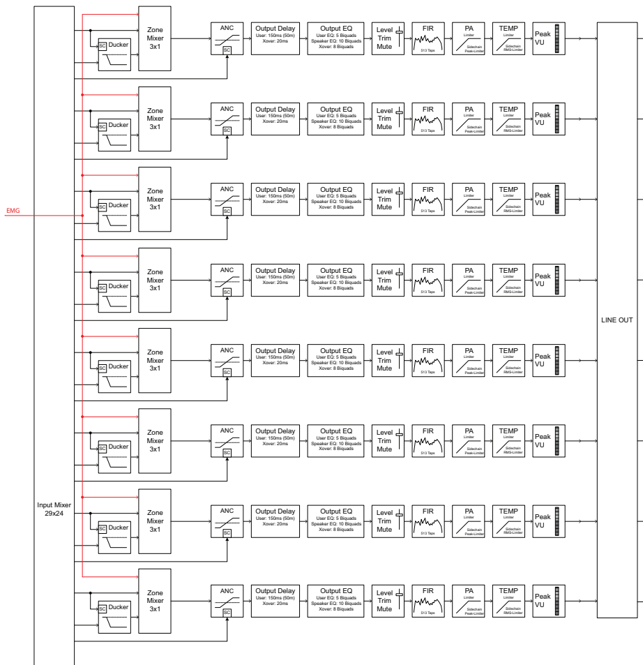
Fig. 3: Salidas DSP
