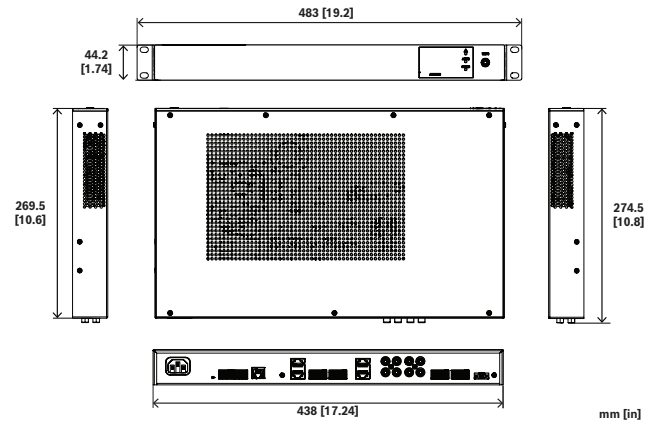
Fig. 1: Dimensions
