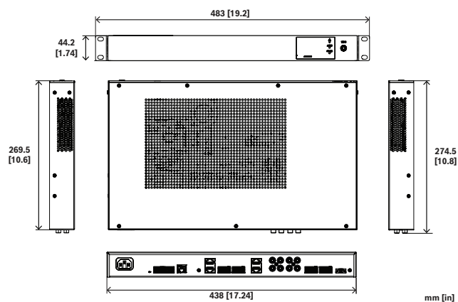
Fig. 1: Dimensioni
