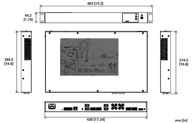
Рис. 1: Габариты
