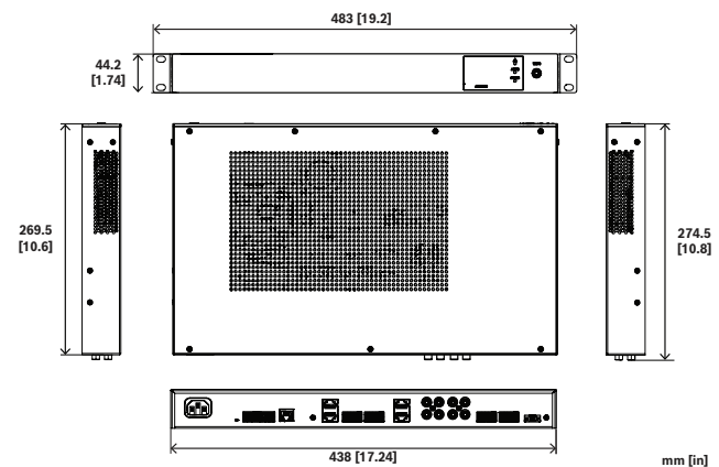
图片 1: 尺寸
