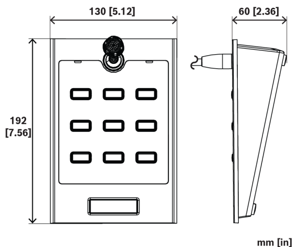
図. 1: 寸法
