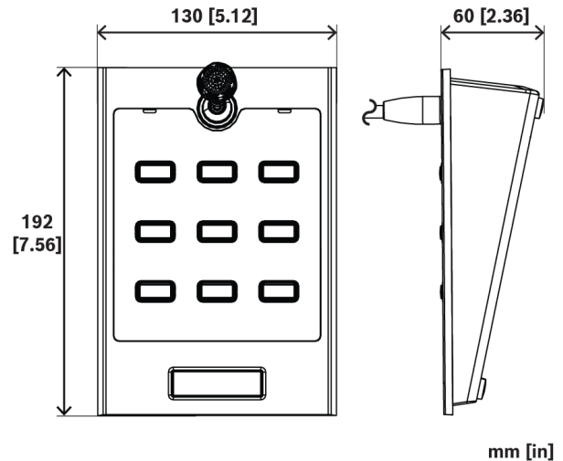
Afb. 1: Afmetingen
