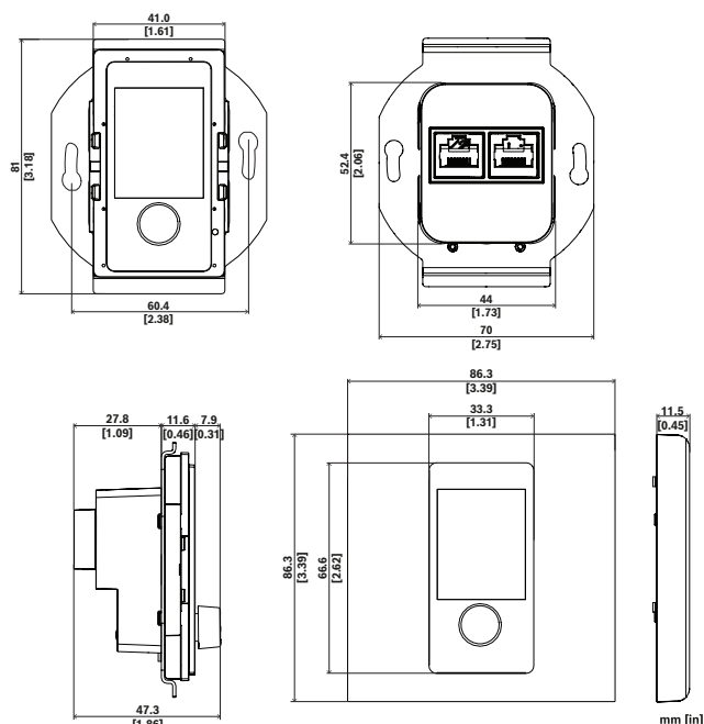
Рис. 1: Габариты
