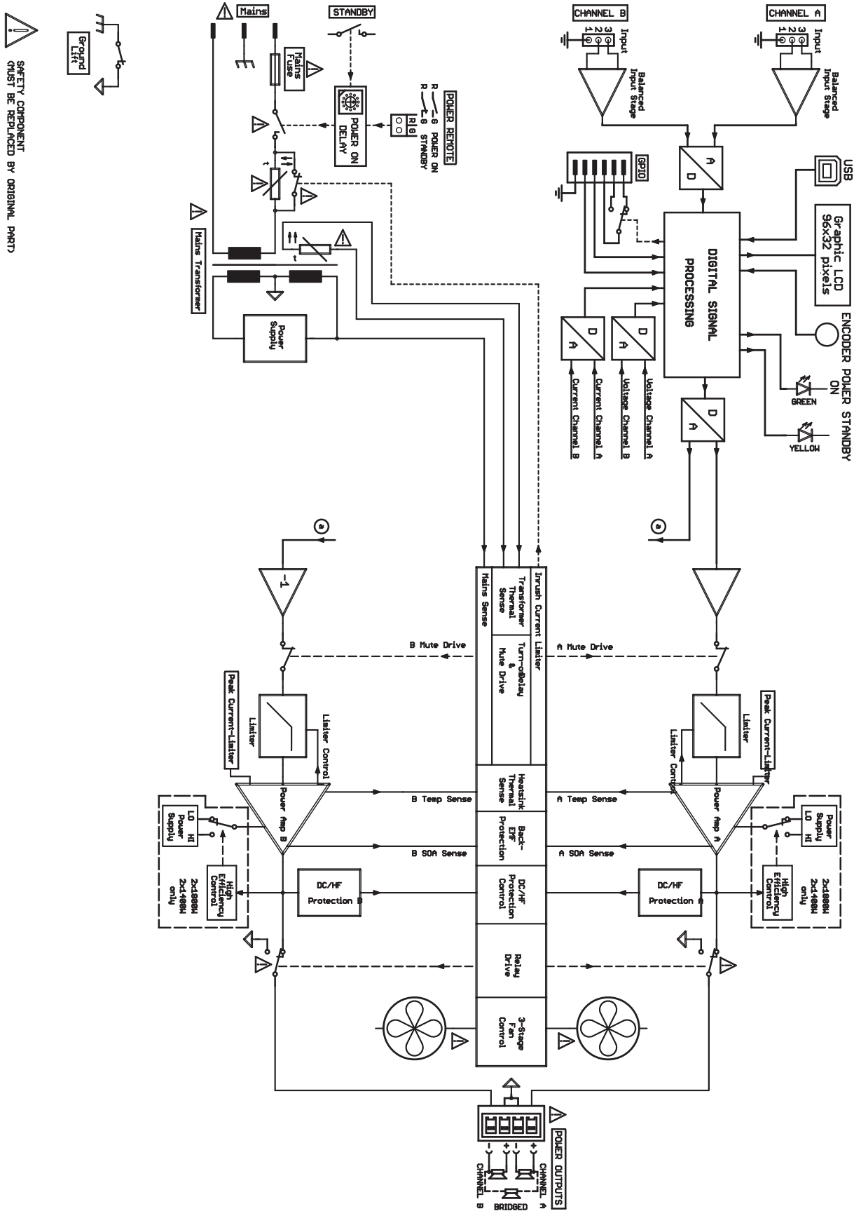
8.2: C シリーズアンプのブロック
