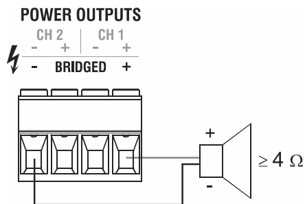
図 6.5: ブリッジモード
