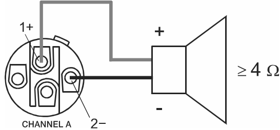
図 6.3: ブリッジモード
