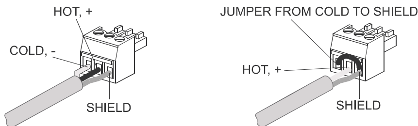
図 6.9: 入力の平衡/不平衡接続
