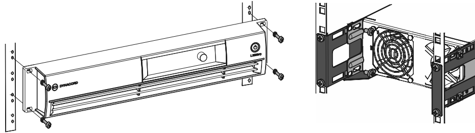
図 5.3: パワーアンプのラックへの取り付け、前面 (左) と背面 (右)、オプションの RMK-15 を示す
