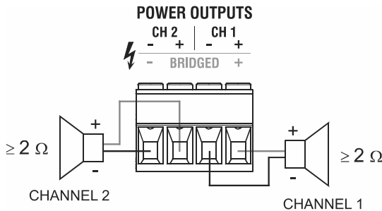
図 6.4: ノーマルモード
