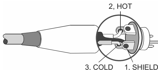
図 6.6: 入力の平衡接続
