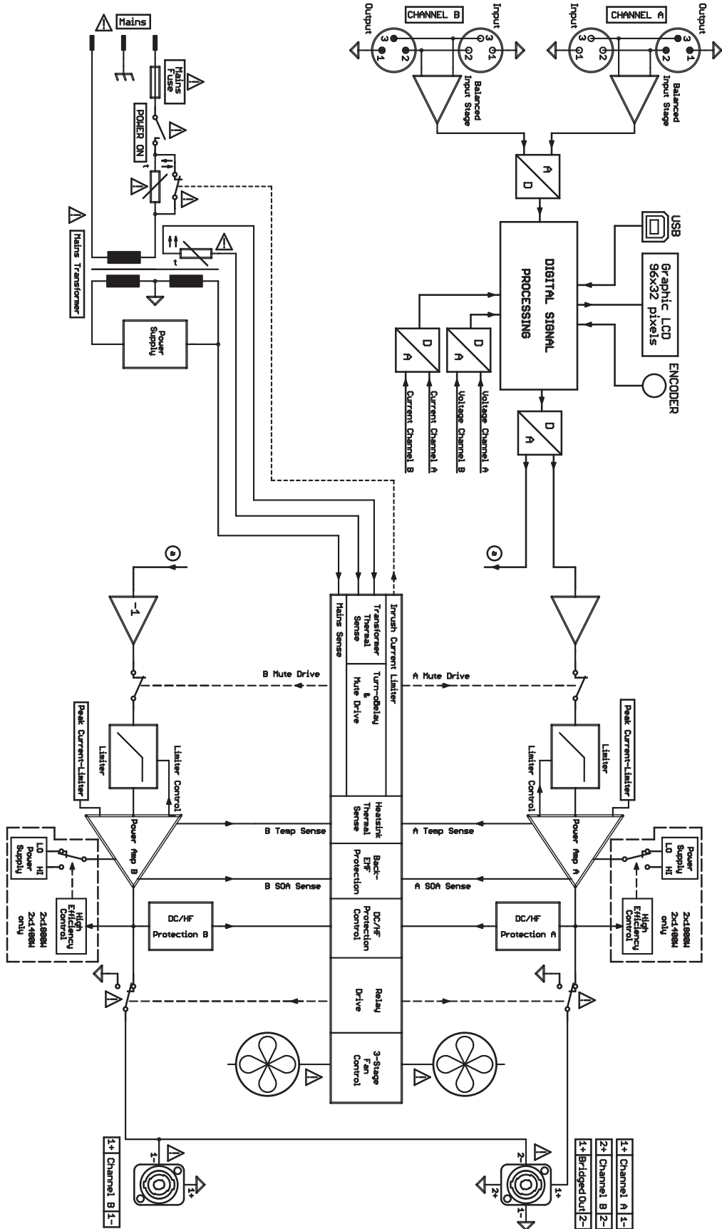
図 8.1: L シリーズアンプのブロック図
