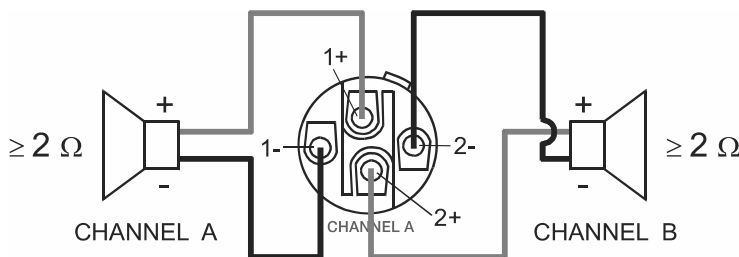
図 6.2: ノーマルモードのバイアンプ配線
