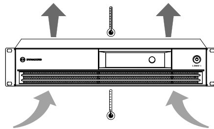
図 5.4: パワーアンプの通気
