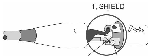
図 6.8: 出力の平衡接続 (デージーチェーン)
