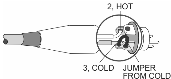
図 6.7: 入力の不平衡接続
