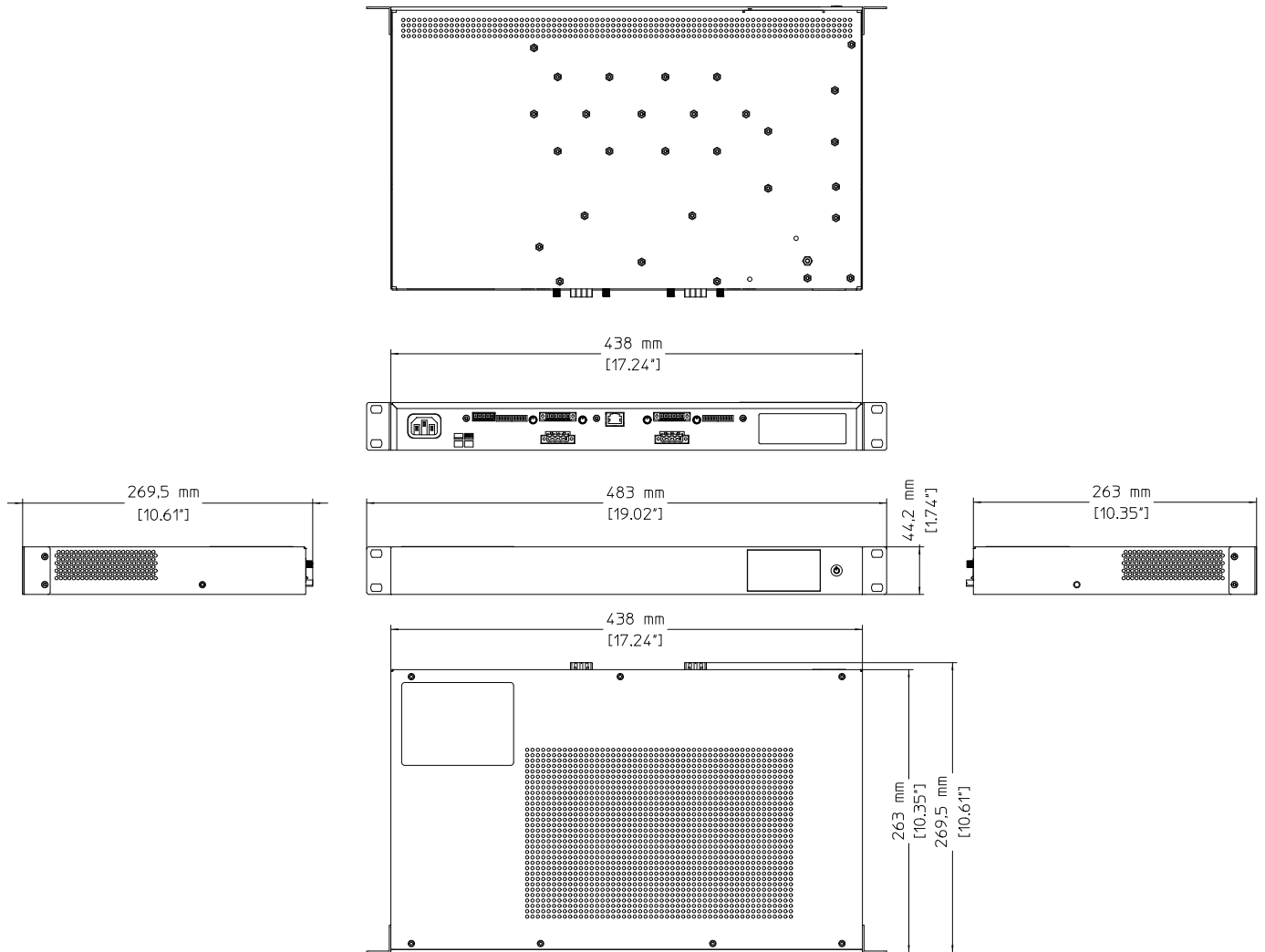
Afb. 3: Afmetingen
