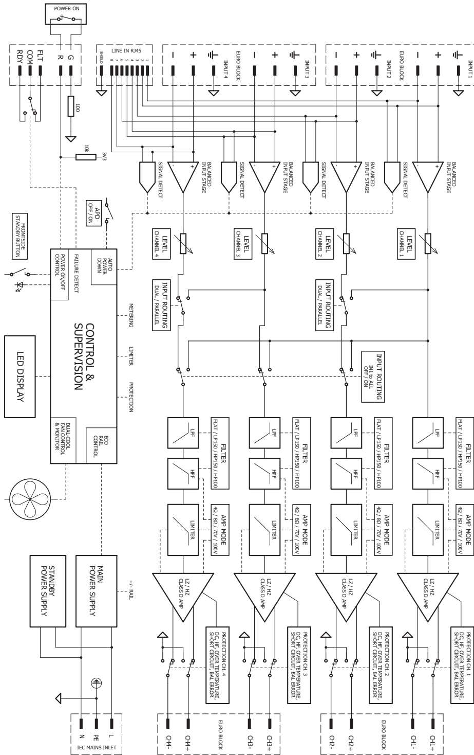
Afb. 2: Blokschema
