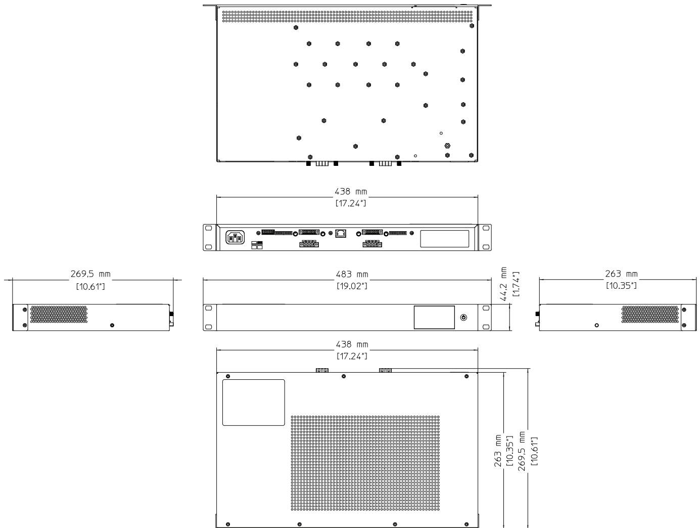
Rys. 3: Wymiary
