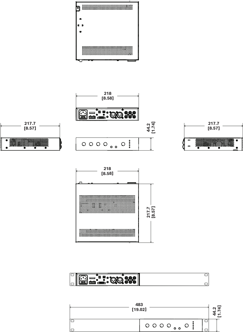
Fig. 1: Dimensiones
