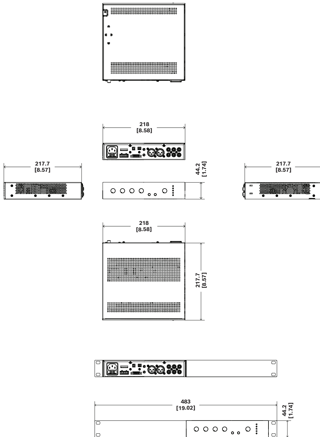
Fig. 1: Dimensions
